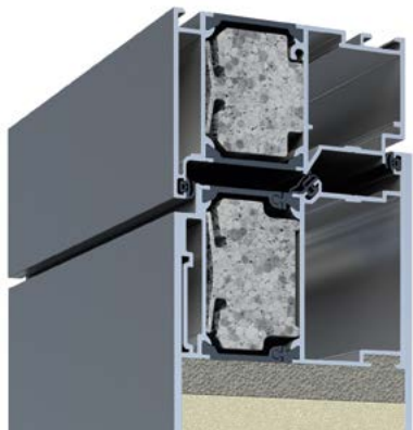
Abb. flügelüberdeckende Füllung innen und außen
