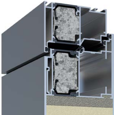
Abb. flügelüberdeckende Füllung innen und außen
